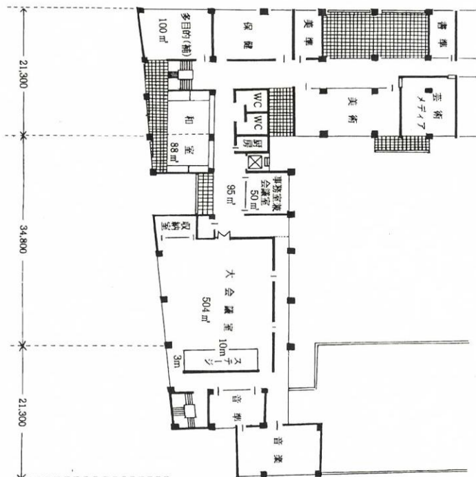
同窓会館平面図 (案)
